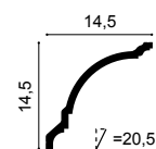
CX203 | CX203F Duropolymer® 200 x 14,5 x 14,5 cm
